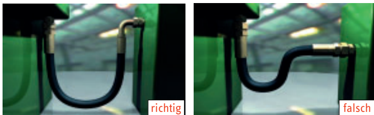
Abbildung 7: Biegeradius
