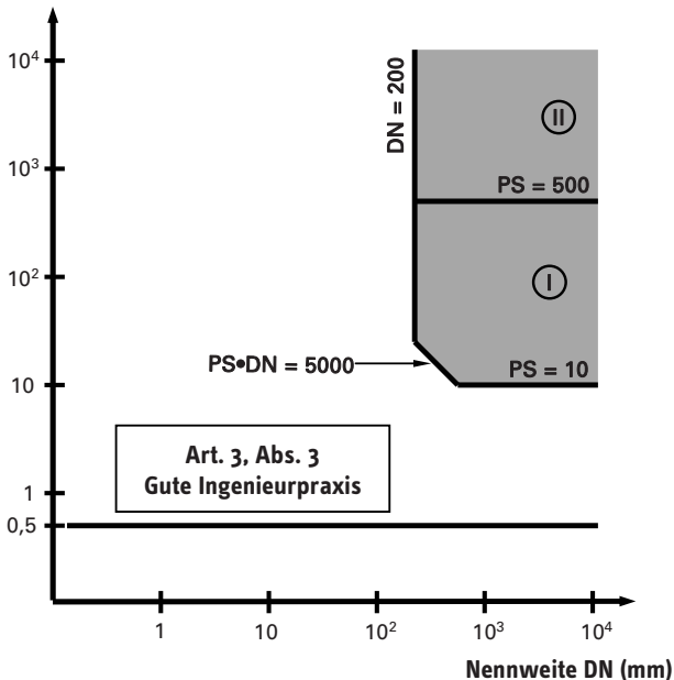
Abbildung 19: Diagramm 9, Anhang II der Druckgeräterichtlinie (Rohrleitungen für Flüssigkeiten der Fluidgruppe 2)
